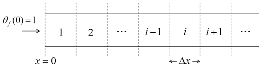
Fig. 3. Discretización del dominio de solución de las ecuaciones (13-15).
